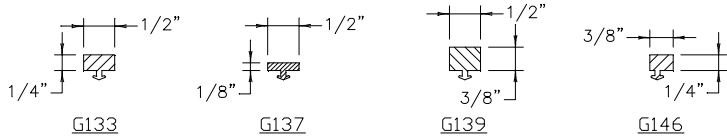
GASKETS
